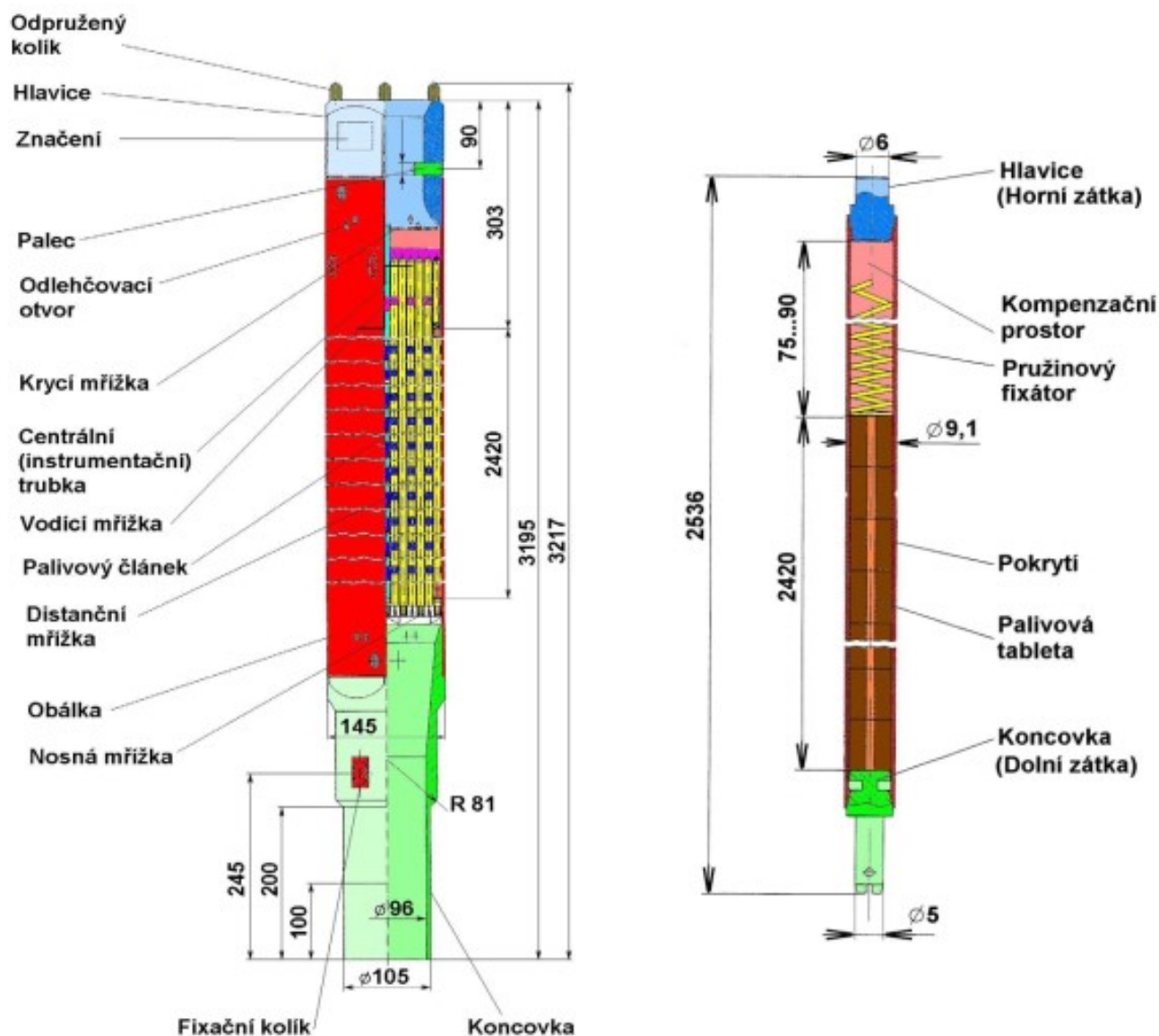
Palivová kazeta s palivem
