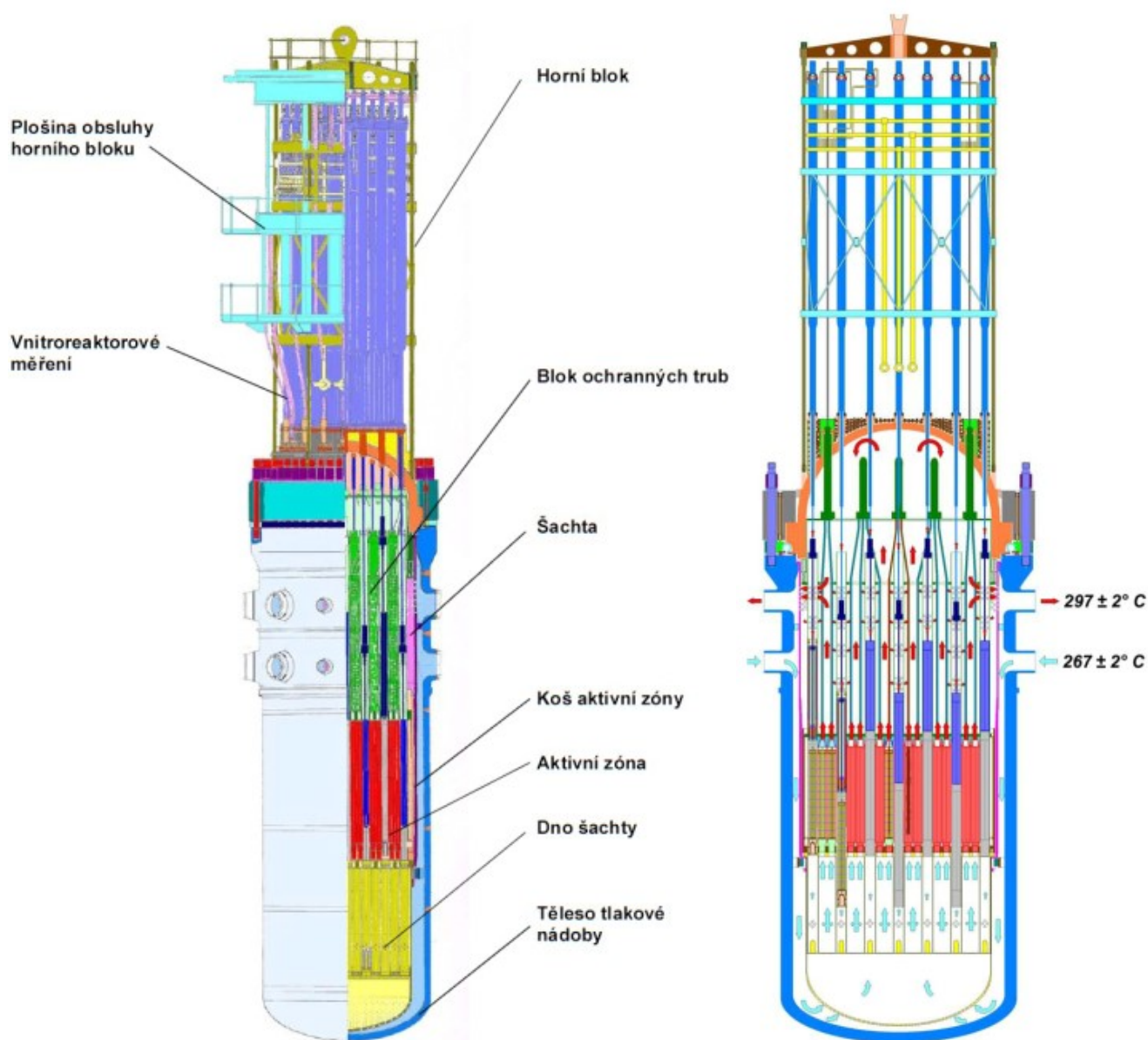
Řez reaktorem VVER 440V
