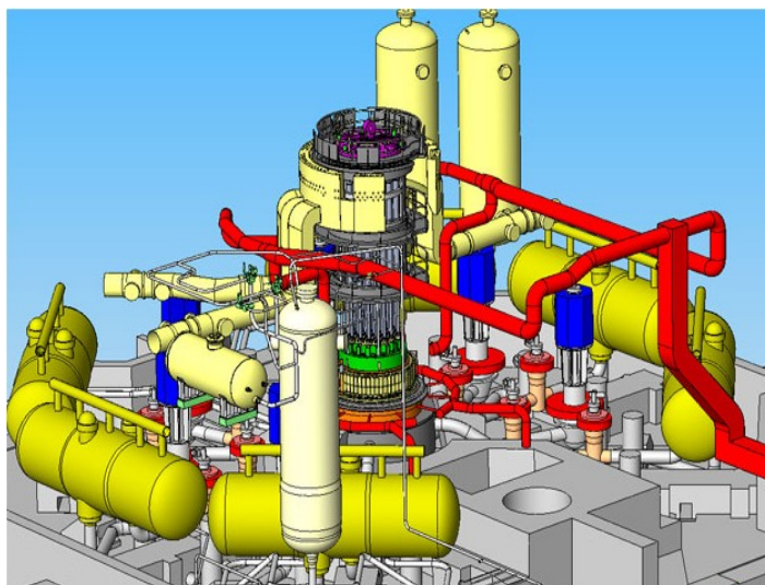
3D schéma uspořádání primárního okruhu
