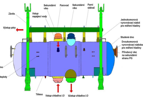
Schéma parogenerátoru
