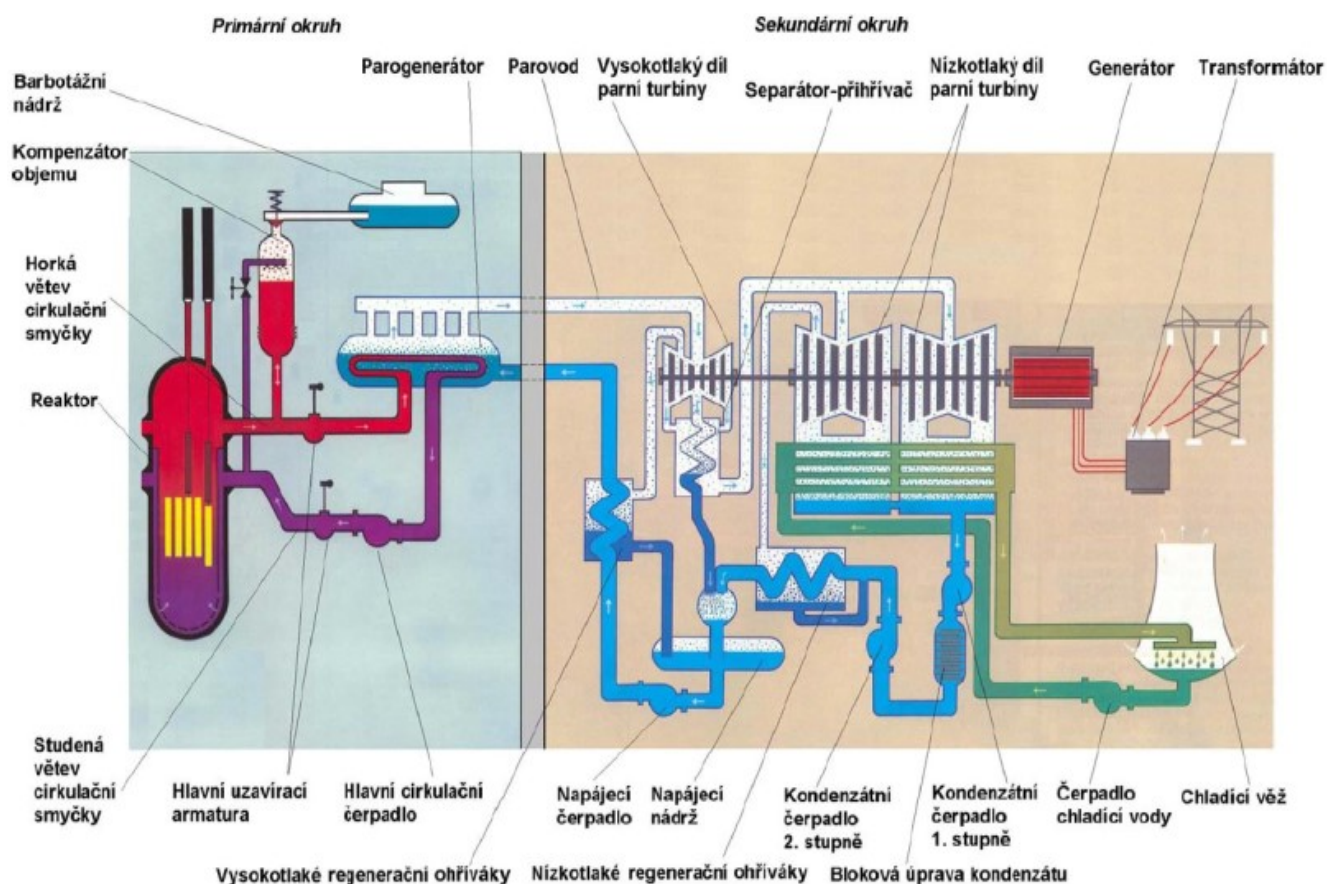
Schéma bloku VVR 500MW v Dukovanech
