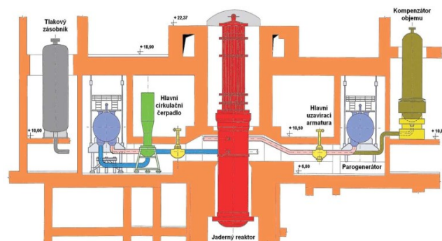
Schéma zapojení reaktoru
