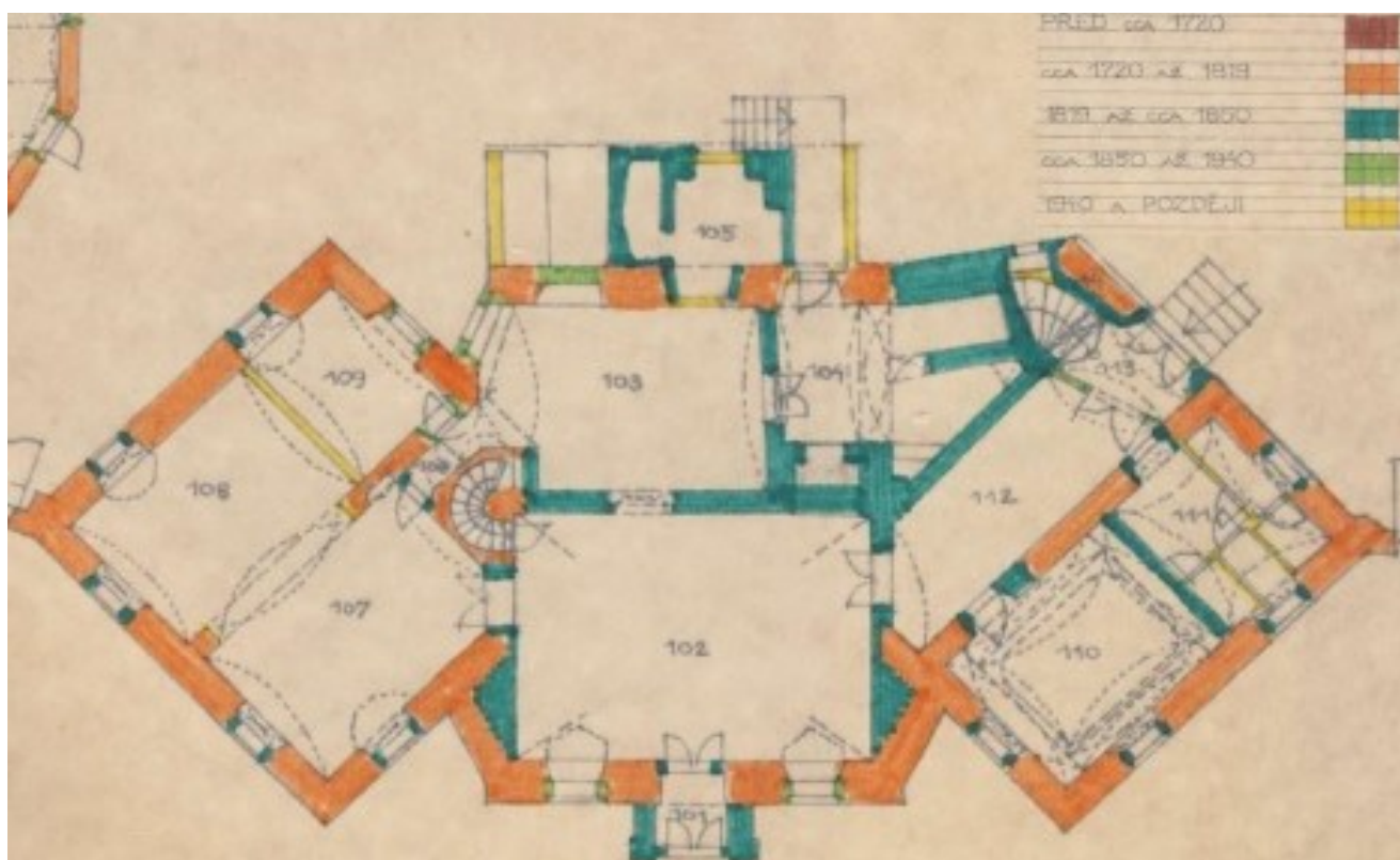
Půdorys stavby
